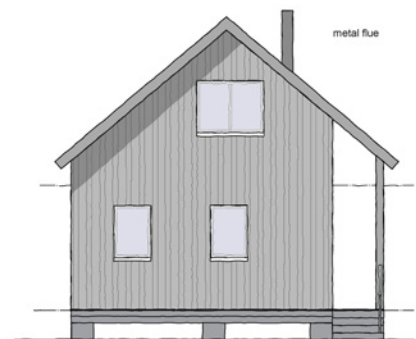
4 Side Elevation Scale: 1:50
