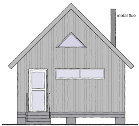
3 Front Elevation Scale: 1:50
