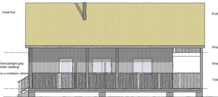
1 Front Elevation Scale: 1:50
