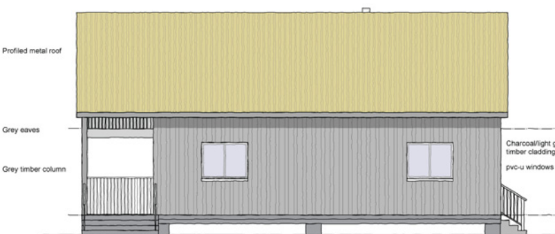
2 Rear Elevation Scale: 1:50
