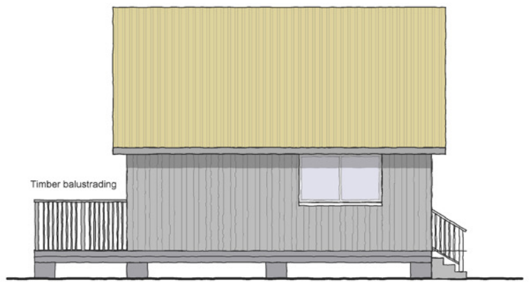
4 Side Elevation Scale: 1:50
